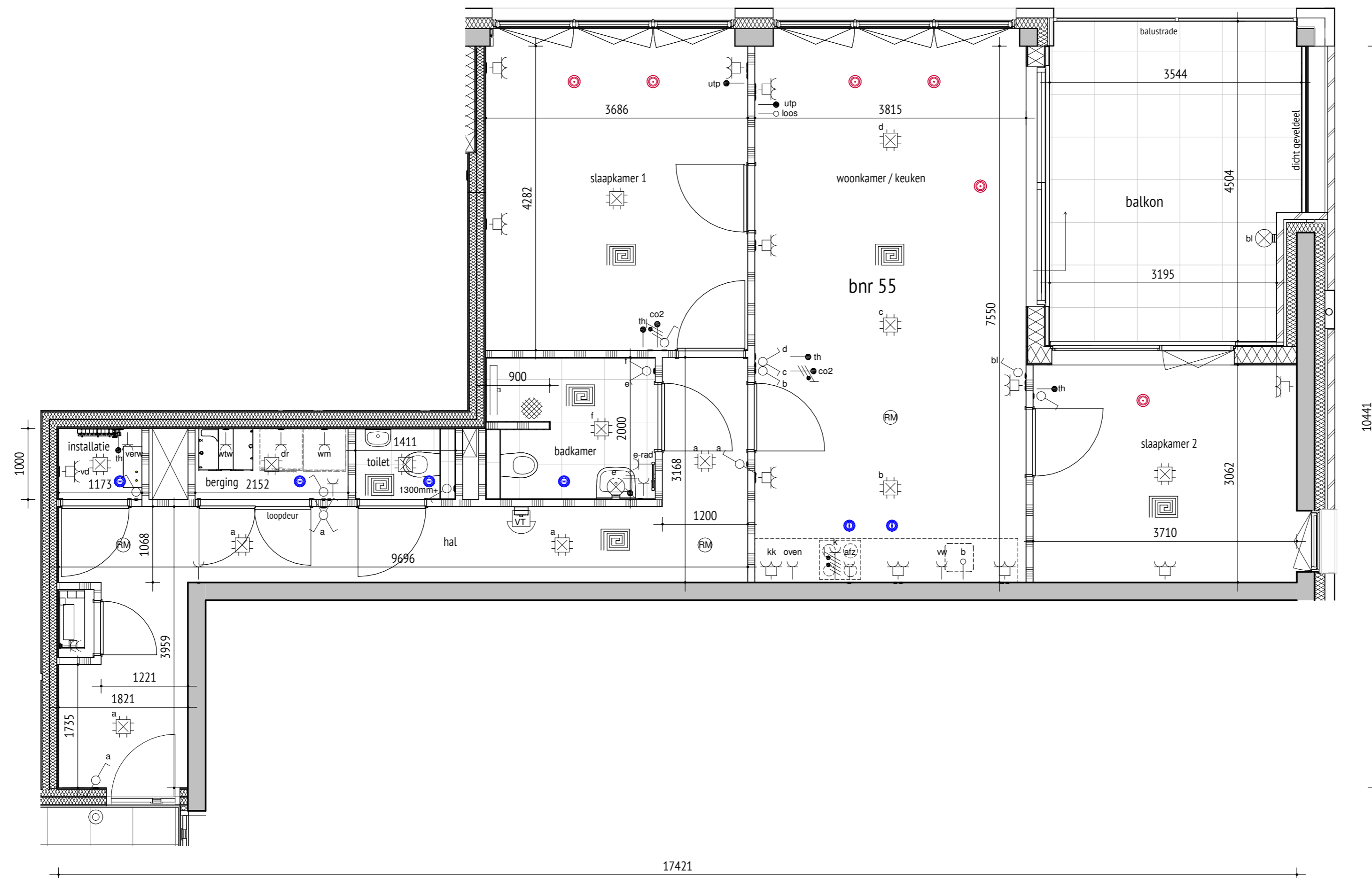
Bnr. 55 - 4de verdieping type C2
