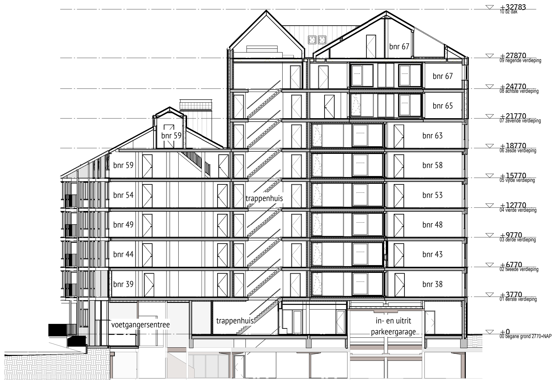
doorsnede AA
